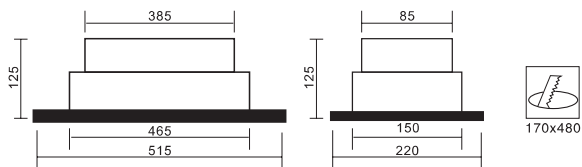
MUA-5023 QR111 50Wx3 G53
