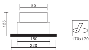
MUA-5021 QR111 50W G53
